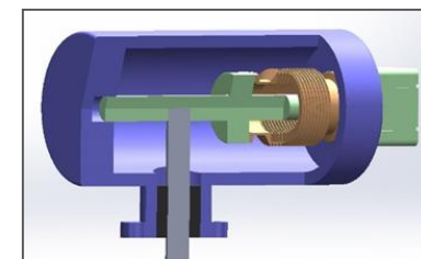
ペローズシール機構
