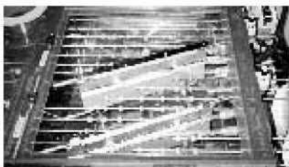
エアークナイフ → Air knife
